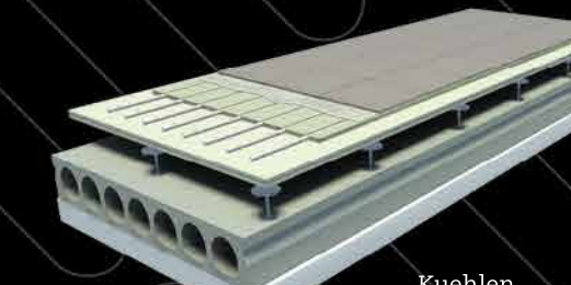
Eingefräste Fußbodenheizung in Knauf Hohlboden mit Fliesen WTP - Nr. 0711002
